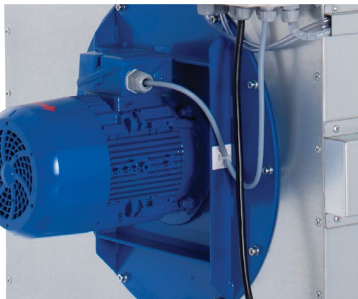
Fig. haut: Vacumobil VT 200 avec un moteur économe en énergie de 4,0 kW (IE3)
